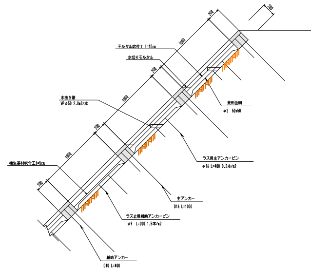
標準断面図 S=1:20
