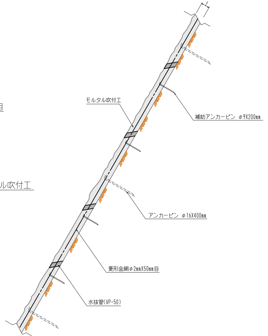
標準断面図
